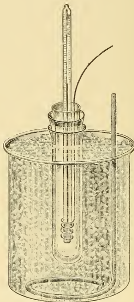
Beckmann's apparatus. (Simon.)
